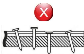
Рис. 3 Пример неправильной забивки гвоздей при монтаже П(Ю)дукции.
