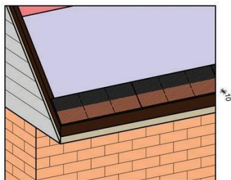
Рис. 11 Схема укладки коньково-карнизной черепицы на карнизе.
