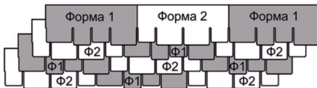
Рис. 15 Схема чередования гонтов гибкой битумной черепицы Döcke PIE коллекции «саппоро».
